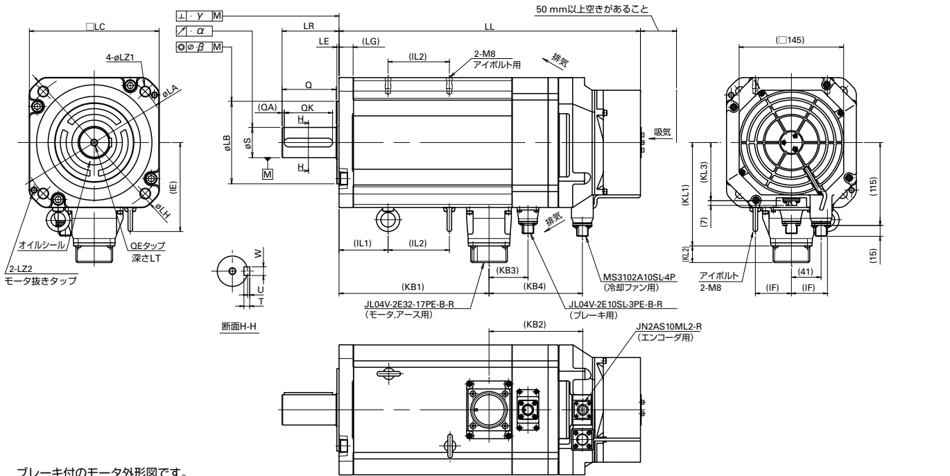
ブレーキ付のモータ外形図です。
