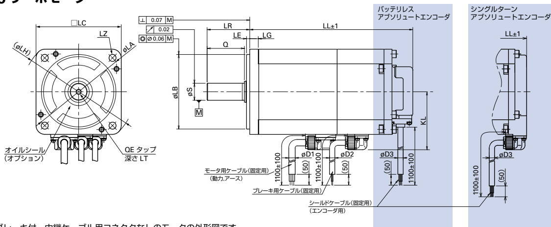
ブレーキ付、中継ケーブル用コネクタなしのモータの外形図です。
