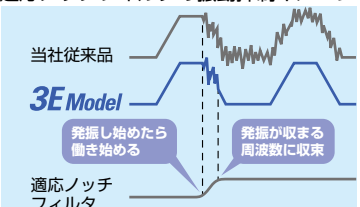
適応ノッチフィルタの振動抑制イメージ
