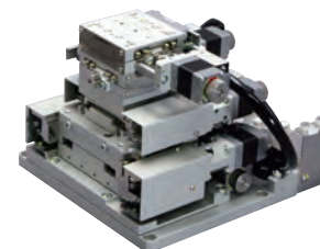
6軸マニピュレータ
