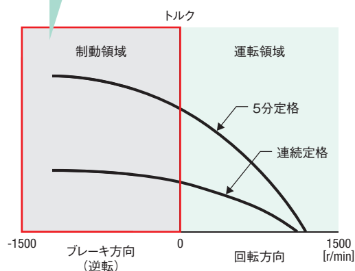
モーターを巻き取り方向と逆回転させます
