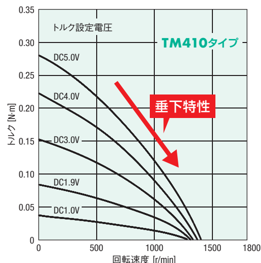
回転速度－トルク特性
