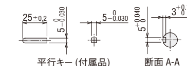
平行キー (付属品)
