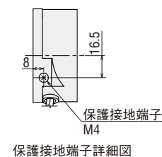
保護接地端子詳細図
