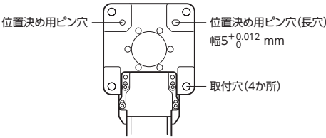
反出力ケーブル側から見た図
