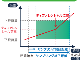
ディファレンシャル荷重(位置)判定・距離指定
