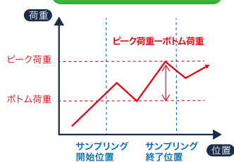
ピークtoピーク荷重判定・位置指定
