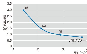
除電時間×風速図(*1)
