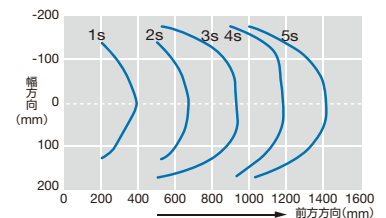
除電領域 — 除電時間特性図(*2)
