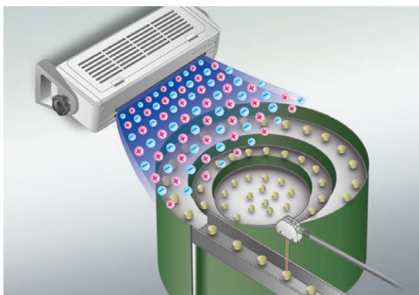
パーツフィーダの除電
