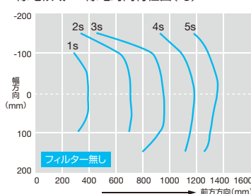
除電領域 — 除電時間特性図（*3）
