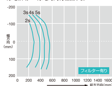
除電領域 — 除電時間特性図（*3）
