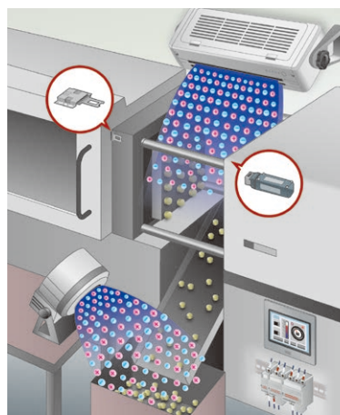
射出成型機、成型部品の除電
