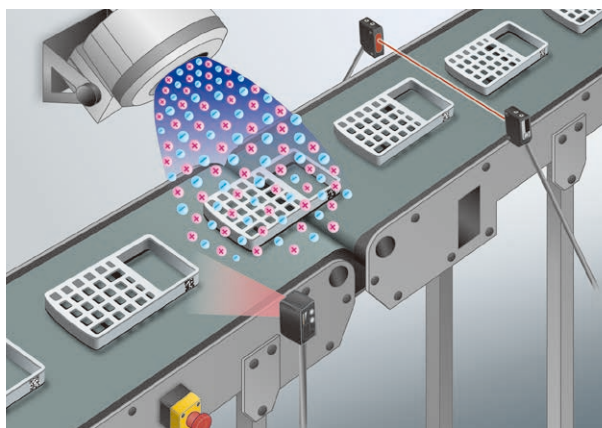
成型部品搬送中の除電
