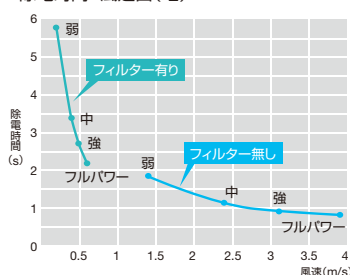
除電時間×風速図（*2）
