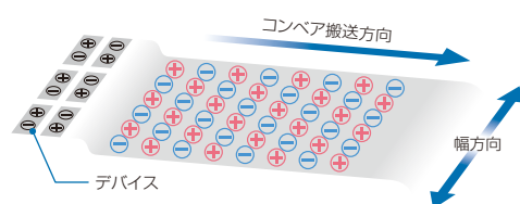
パラレルパルスDC方式(当社)
