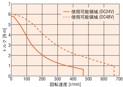
減速比7
