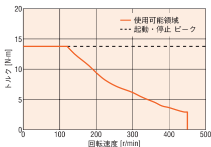
減速比10
