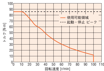
減速比 45
