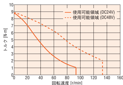
減速比45
