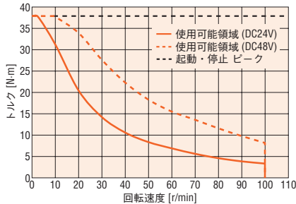
減速比20
