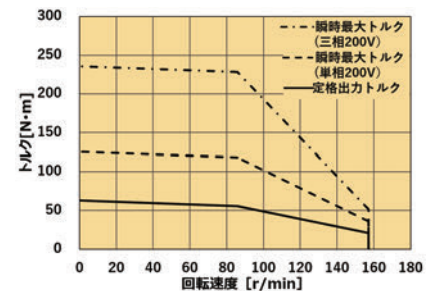
減速比 35
