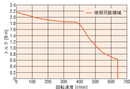
減速比20
