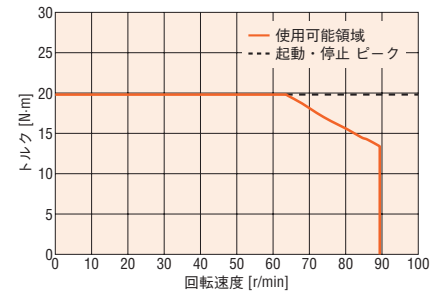
減速比50
