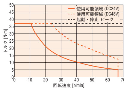
減速比45
