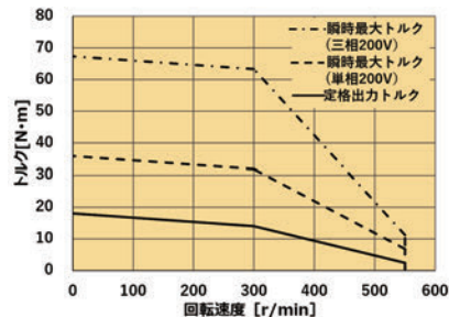
減速比 25
