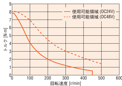
減速比10
