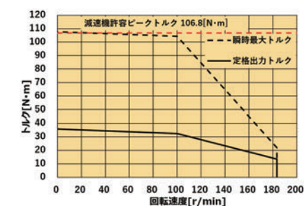
減速比 30
