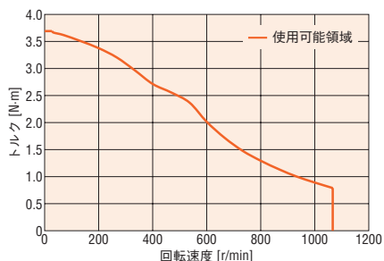
減速比 7
