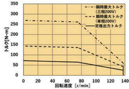
減速比 40
