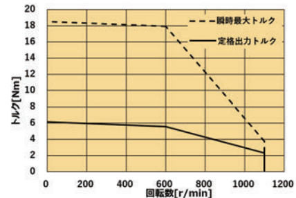
減速比5
