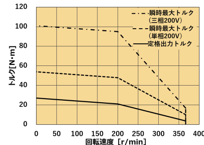
減速比 30
