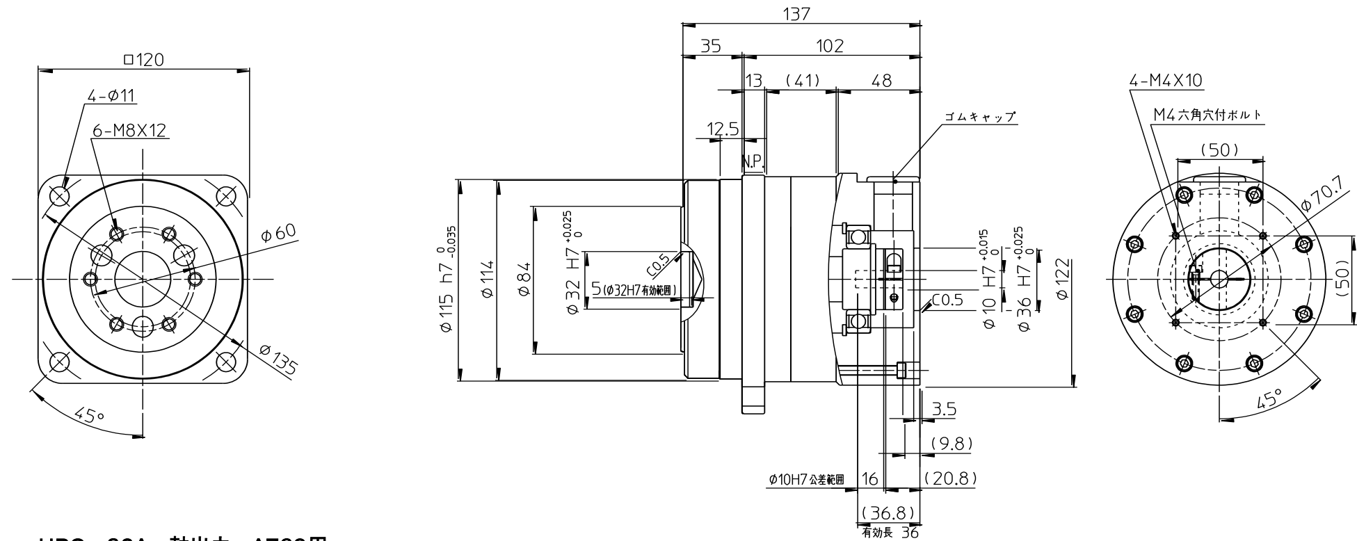
HPG-32A-軸出力-AZ69用
