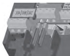
ツイン端子使用例
