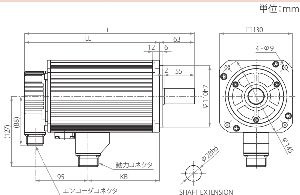
GYS モータ (ブレーキ付)
