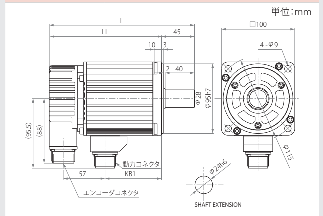
GYS モータ (ブレーキ無)
