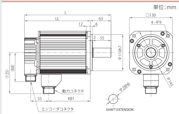
GYS モータ (ブレーキ無)
