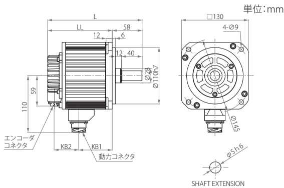
GYG モータ (ブレーキ無)
