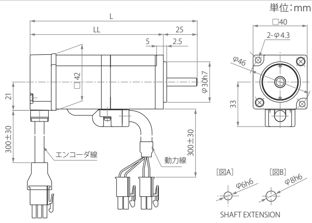
GYS モータ (ブレーキ付)
