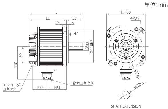
GYG モータ (ブレーキ無)
