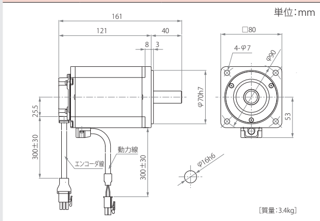
GYS モータ (ブレーキ無)
