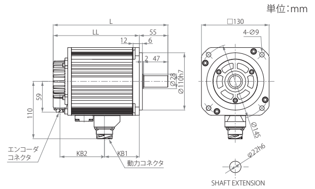
GYG モータ (ブレーキ付)
