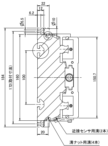
【A-A 断面】
