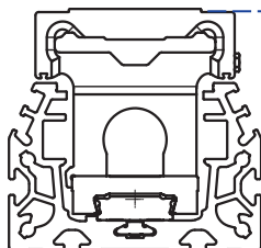
【ELGA-BS】
