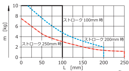
EGSL-BS-55
