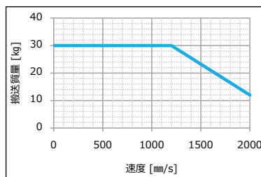
ELGR-TB-55
