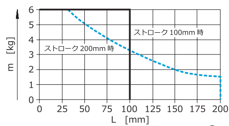
EGSL-BS-45
