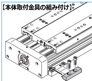
【本体取付金具の組み付け】
