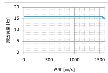
ELGG-TB-45※5
