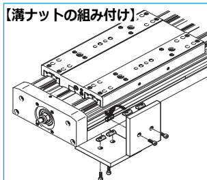
【溝ナットの組み付け】
