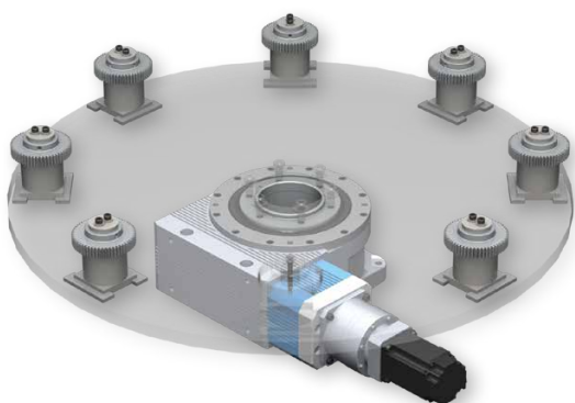
インデックステーブル
