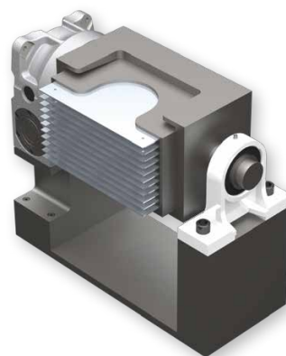
ゆりかご駆動
