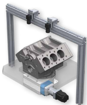
ワークポジショナ
